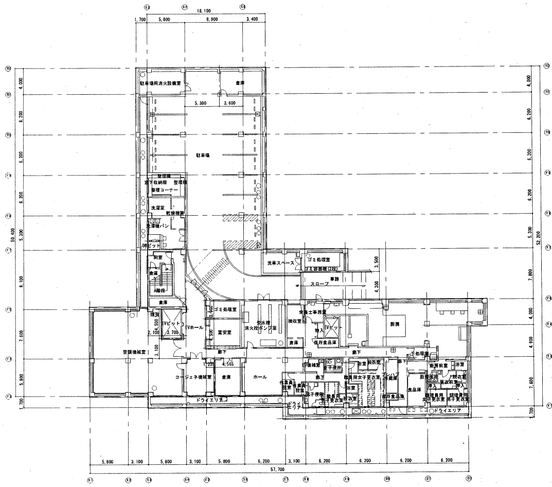
地下1階平面図 S=1/200
