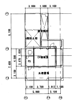
PH2階平面図 S=1/200
