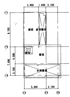
R階平面図 S=1/200
