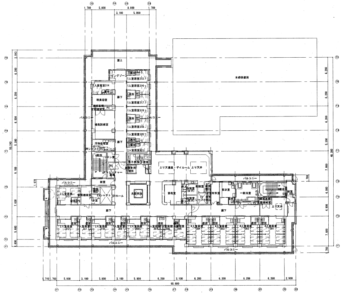
3階平面図 S=1/200
