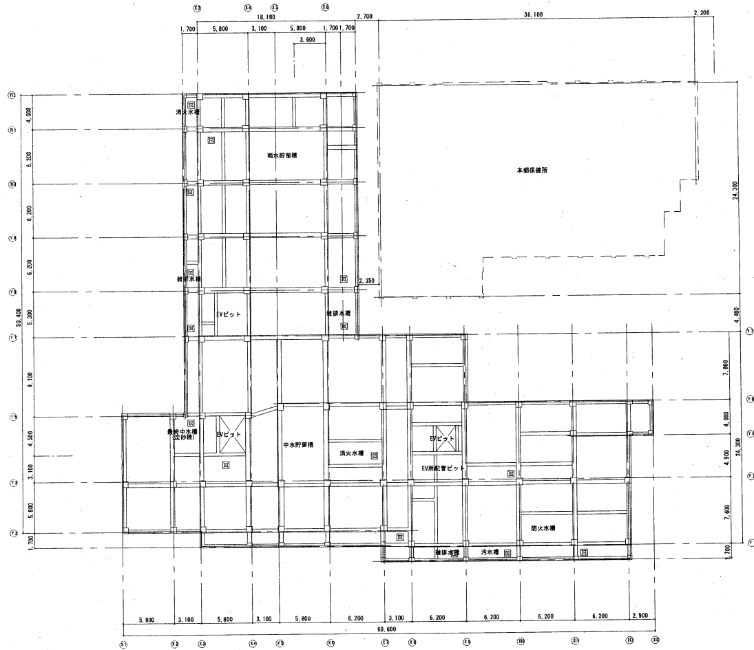
ピット平面図 S=1/200
