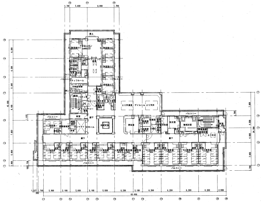
4階平面図 S=1/200
