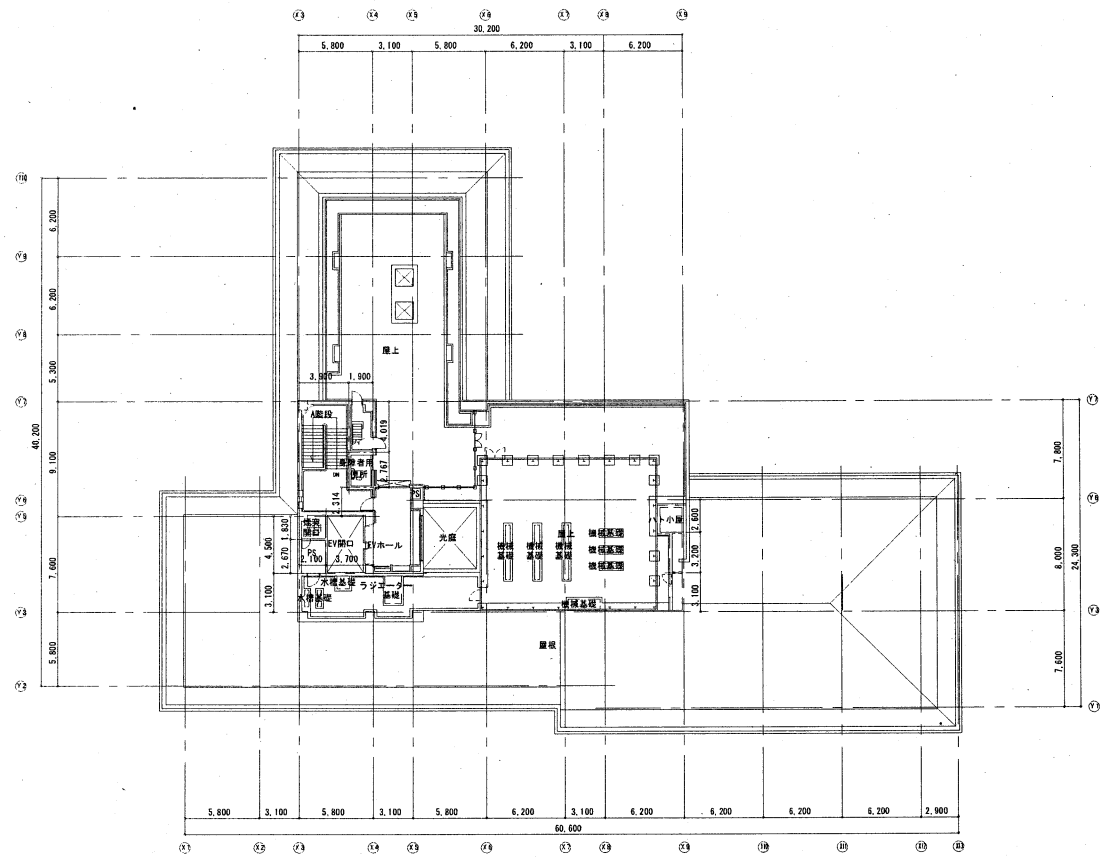
PH1階平面図 S=1/200
