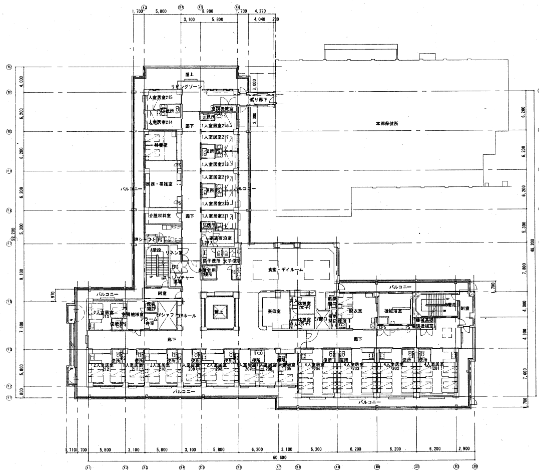
2階平面図 S=1/200
