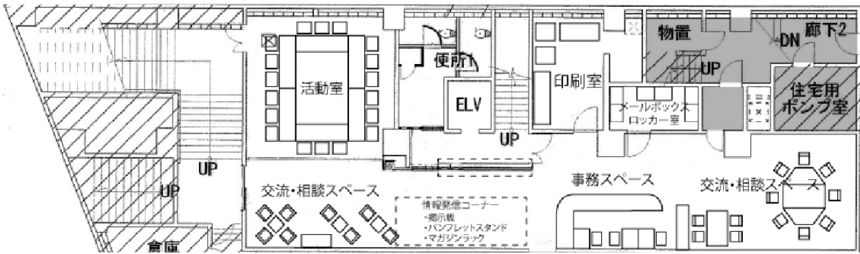
[区民センター地下1階のレイアウト平面図]
