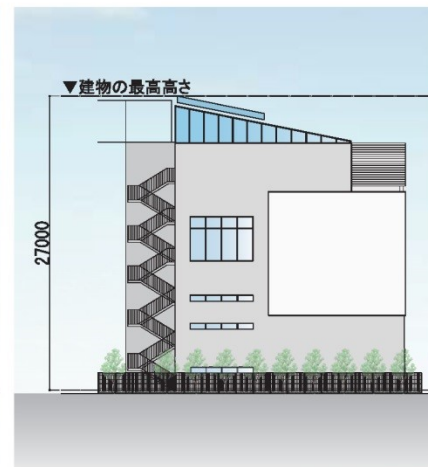
南側立面図
