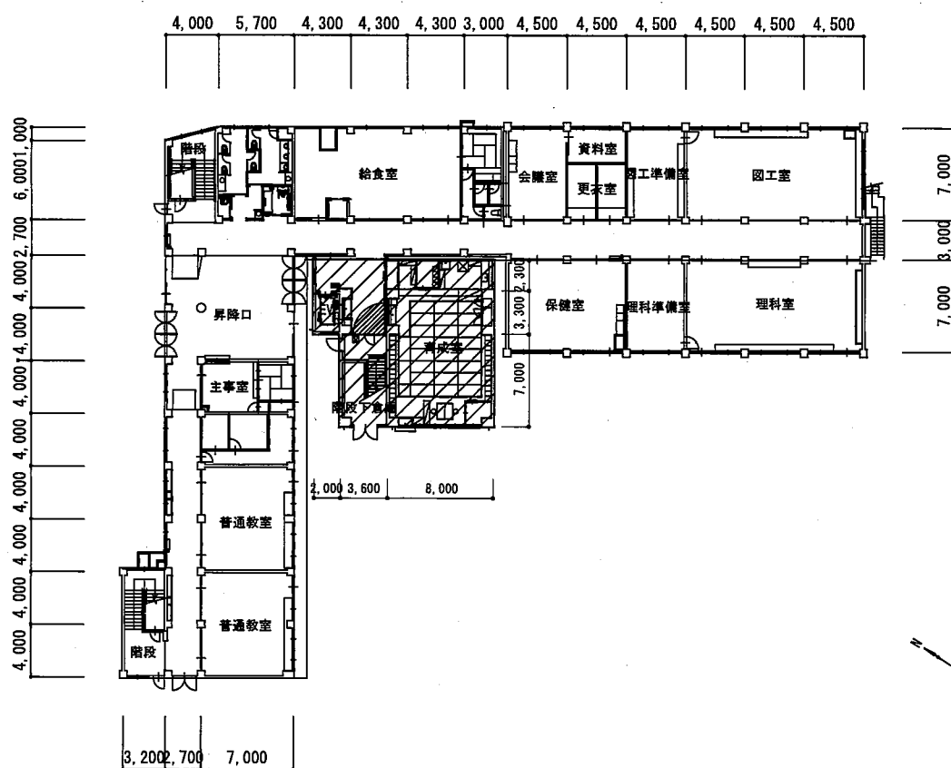
1 階平面図
