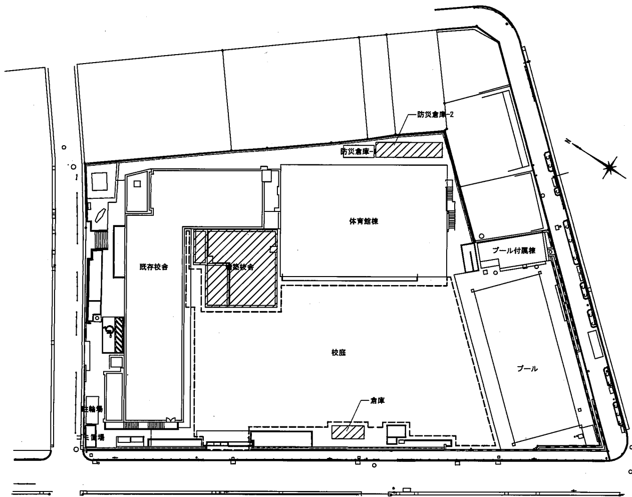
増築配置図 S=1/600
