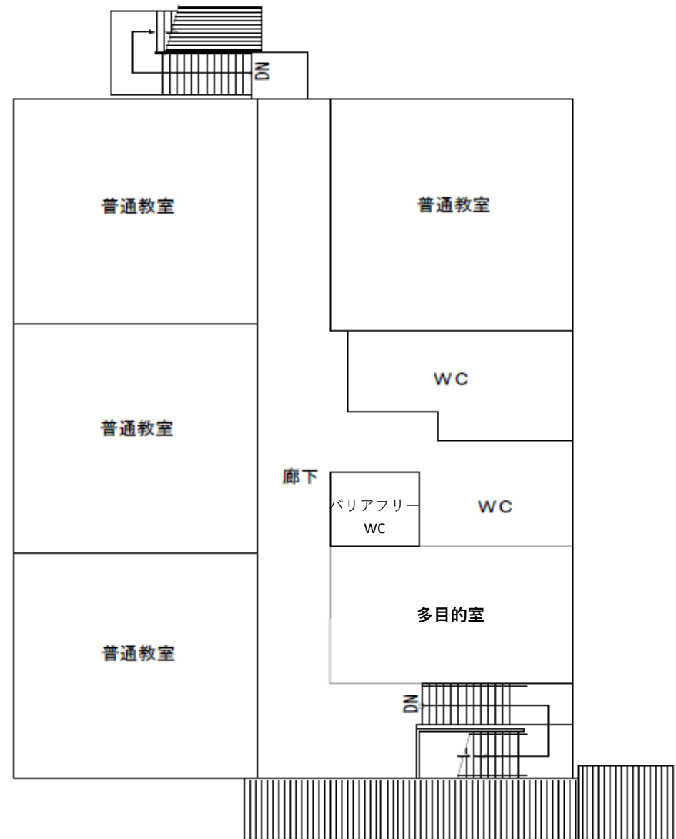
2階平面図
