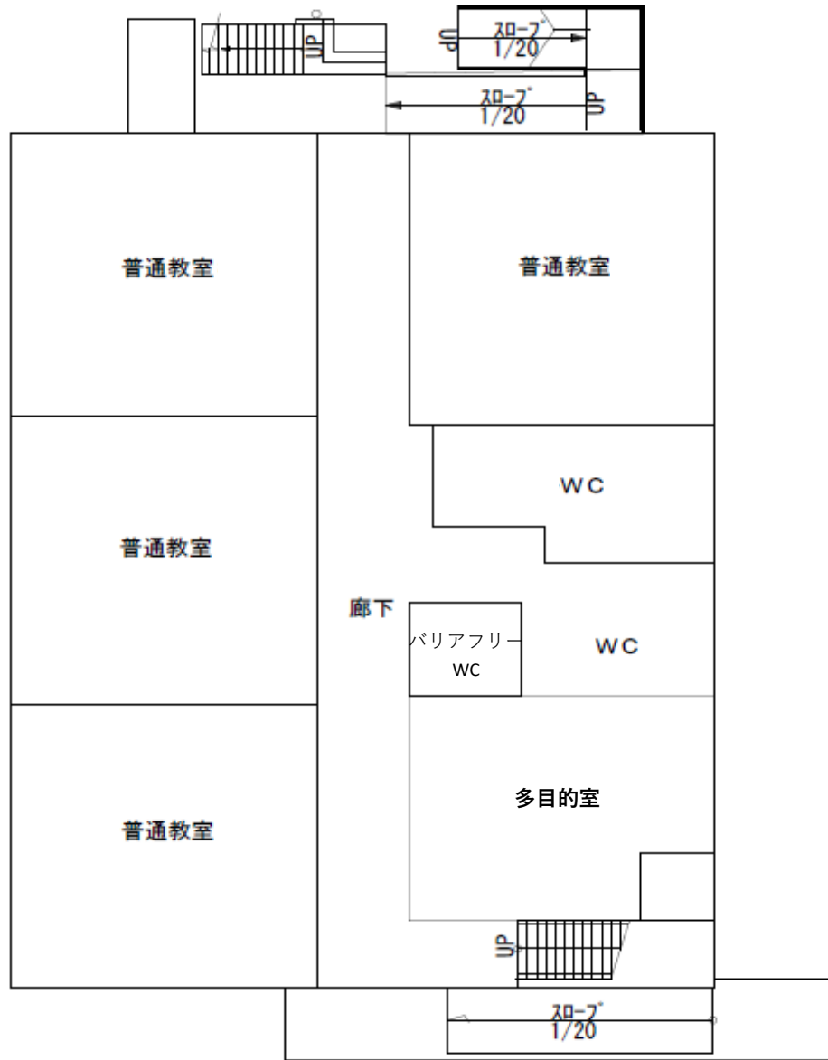
1階平面図
